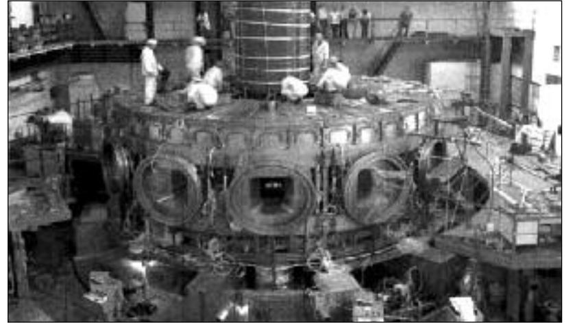
Termodjaderný reaktor Tomakak T15 MD v Institutu Kurčatova v Moskvě
